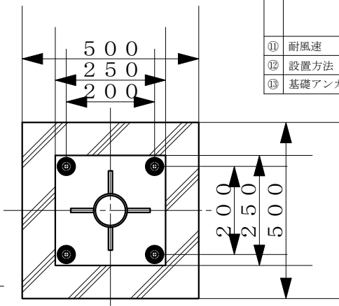
A~A 矢視 S=1/12
